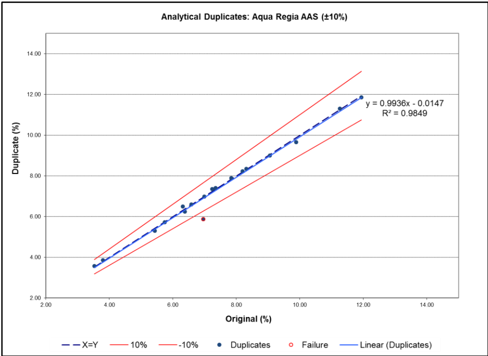
Figure 11-36: Linear Regression of Aqua Regia AAS Manganese Analytical Duplicates Source: Tetra Tech (2022)
