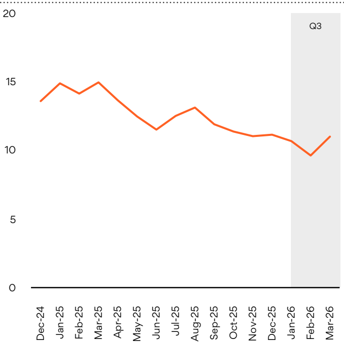
JKM (US$/mmbtu)
